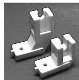
A832 (per cerniere invisibili) A832SD c/salvadito A832E economico A832B gambo basso in plastica (S518) A832A A832ASD c/salvadito A832AE economico (S518N) A832P gambo alto plastica A832PB gambo basso Per cerniere invisibili in materiale plastico per mc/domestiche A832AP gambo alto plastica A832APB gambo basso
